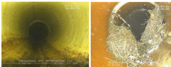
Anschlussleitung Hs.Nr. 6
